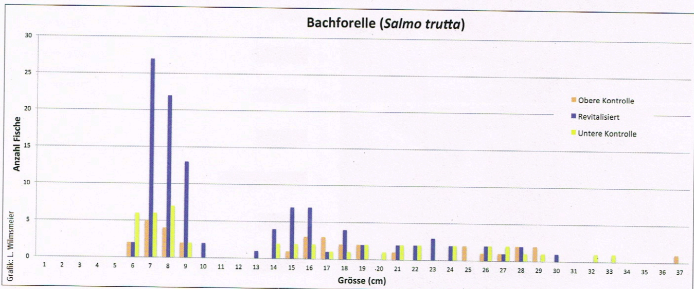
▼ Abbildung 2: Anzahl Forellen bestimmter Grössen in den verschiedenen Abschnitten des Mungnaukanals. Die Abgrenzung der 0+-Fische ist durch die deutliche Lücke (keine Fische mit 11 oder 12 cm Länge) eindeutig möglich.
